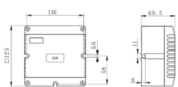
Size 2 CZ0520/□-31
