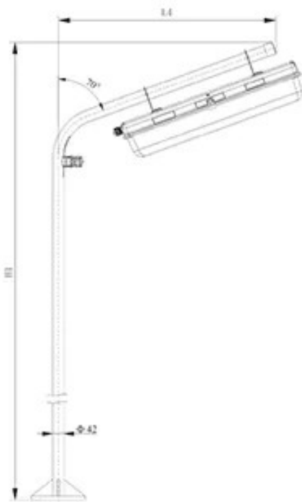
法兰式安装
