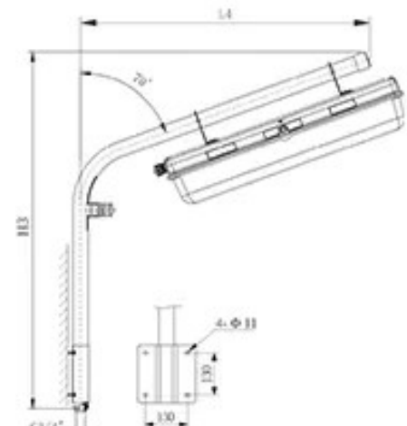
壁式安装
