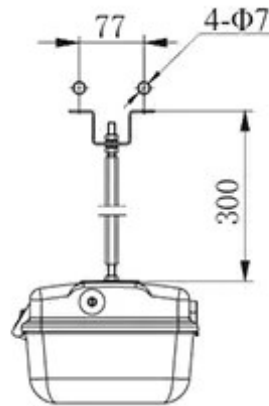
Pendant type
