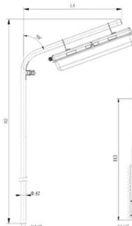
护栏式安装
