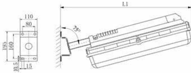
全塑防爆(应急)条形灯(杆式安装)
