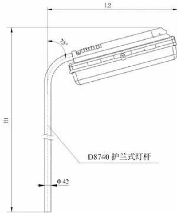
护栏式安装
