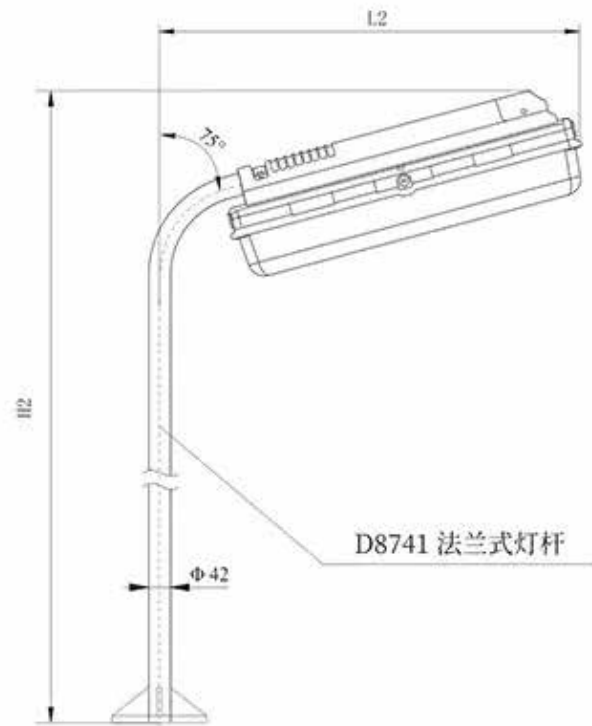
法兰式安装
