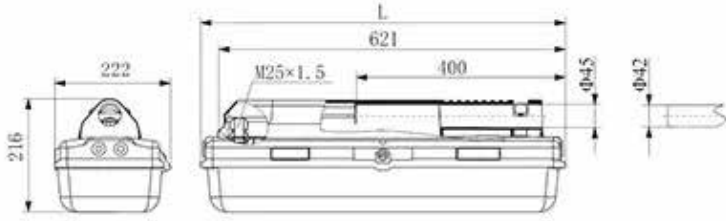
全塑防爆(应急)条形灯(杆式安装)
